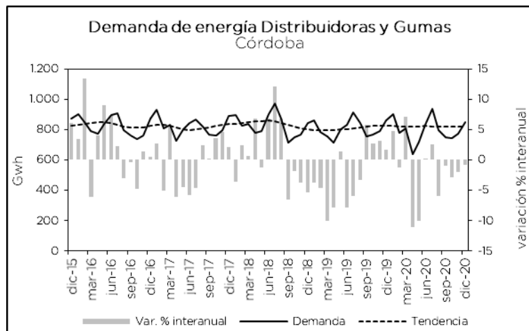
Demanda de energía eléctrica GUMAs por sector Córdoba - Gwh
